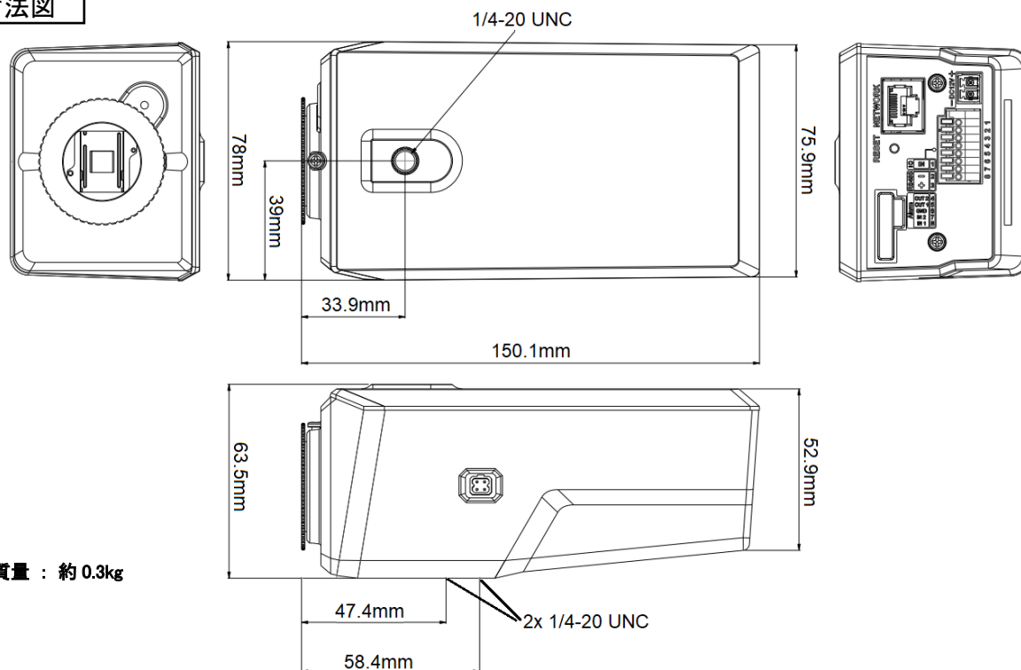
寸法図
